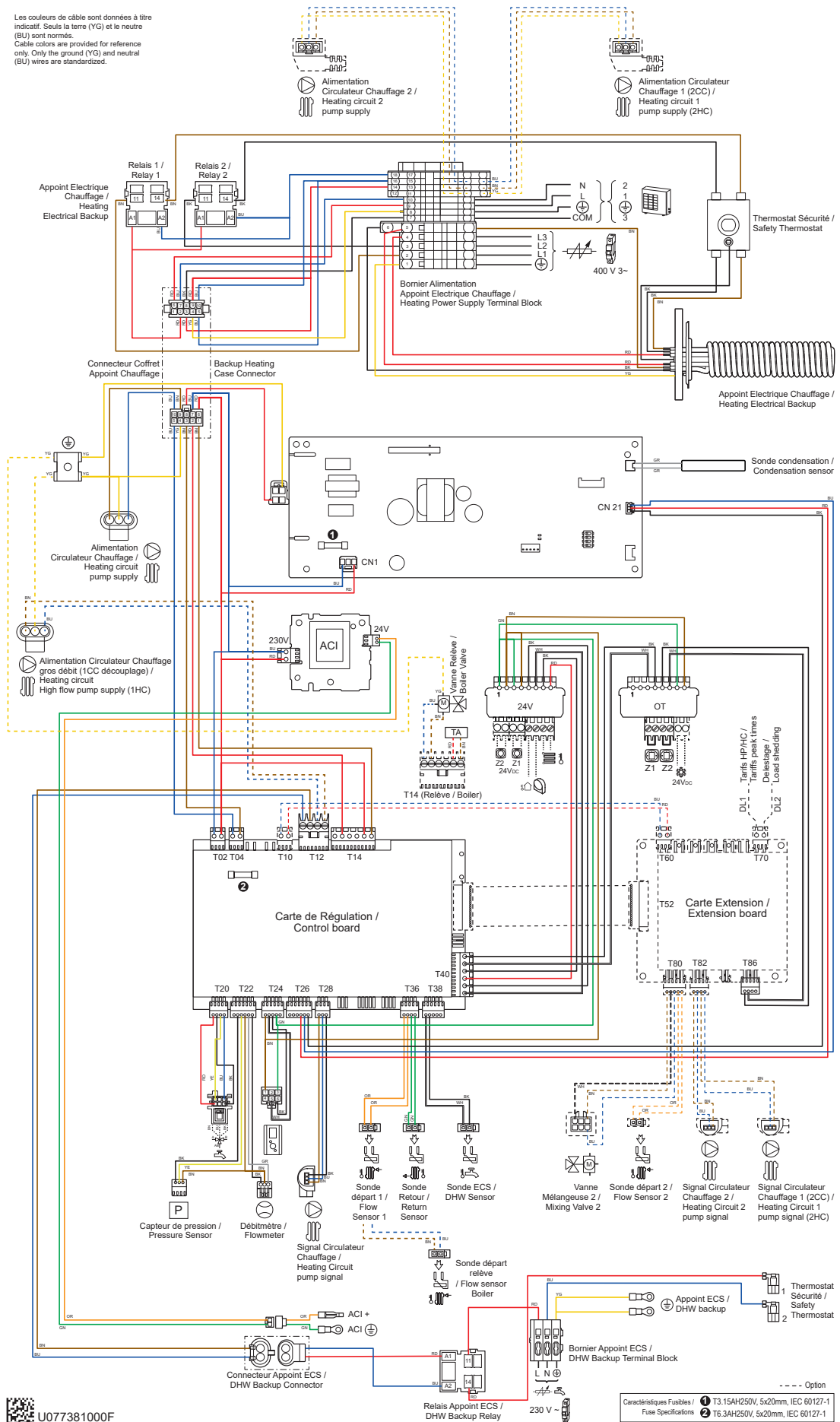
fig. 48 - Câblage électrique du Module Hydraulique - Modèle triphasé
