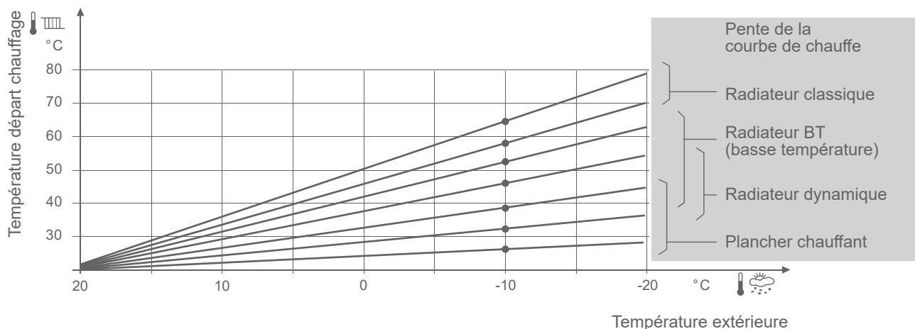
fig. 43 - Pente de la courbe de chauffe
